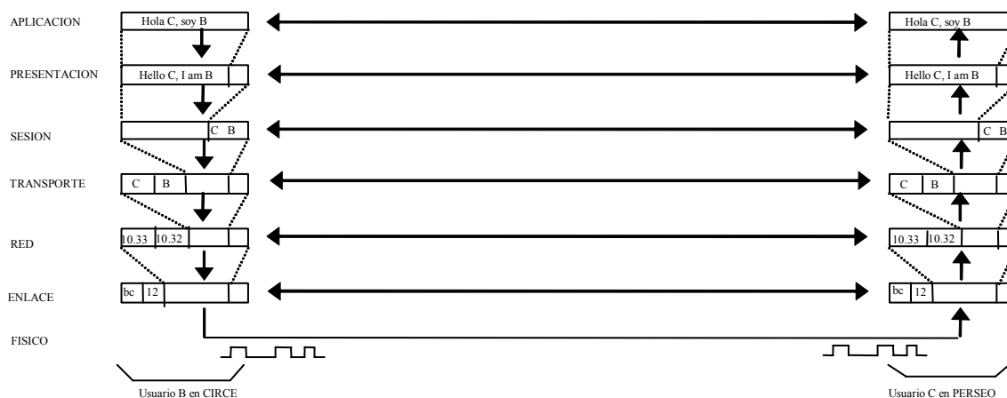
Fig. 12: Ejemplo de comunicación dentro de una subred
