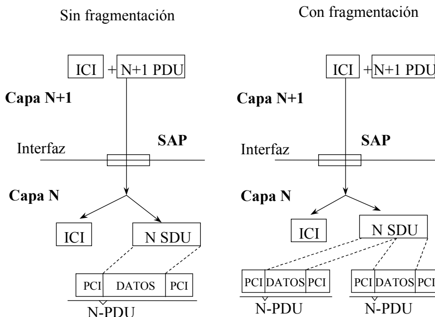
Fig. 6: Uso de los puntos de acceso al servicio
