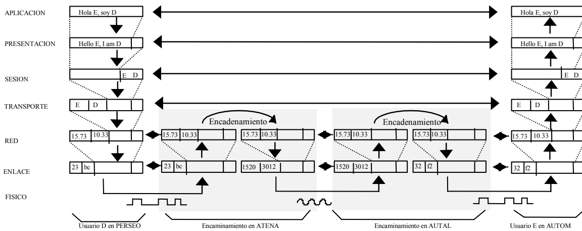
Fig. 13: Ejemplo de comunicación entre subredes
