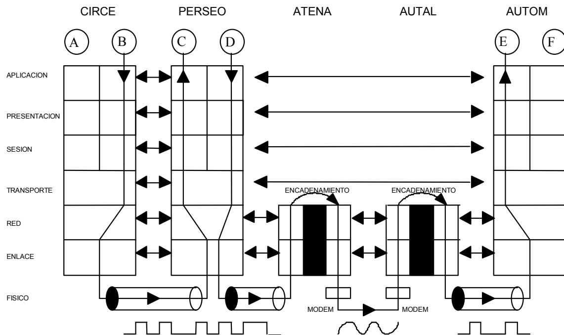
Fig. 14: Representación en el modelo de capas de los ejemplos
