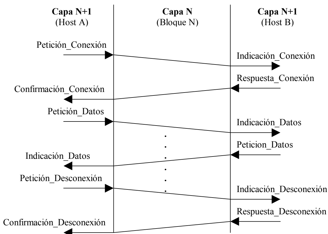
Fig. 8: Servicio orientado a conexión en la Capa N.
